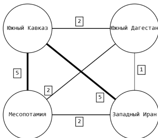
Рис. 3 – Сетевая модель ирано-турецких войн
